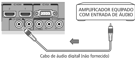
Painel Traseiro do TV
