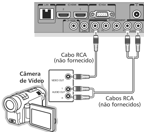
Painel Traseiro Inferior do TV
