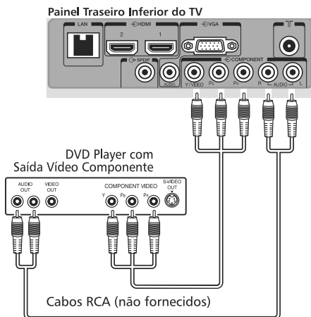
Painel Traseiro do TV
