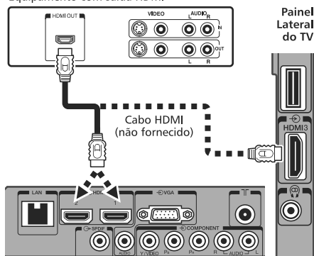
Panel Traseiro Inferior do TV
