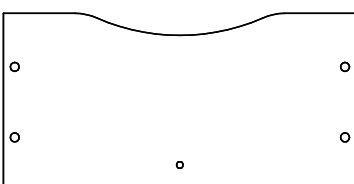
7 (15 x 159 x 320mm) - 3x (0,59 x 6,26 x 12,60in)
