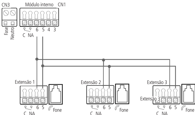
Conexão das extensões de áudio
