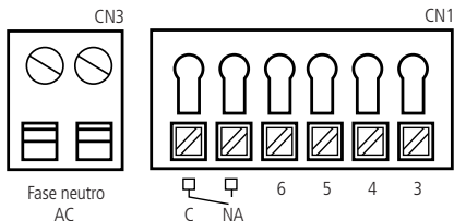
Conectores del módulo interno (MI)
