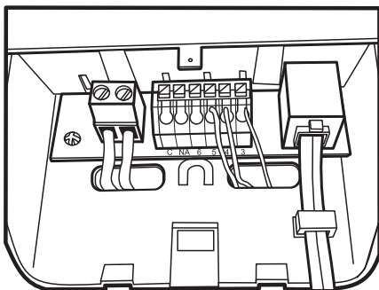
Conexiones de cables en el módulo interno (MI)
